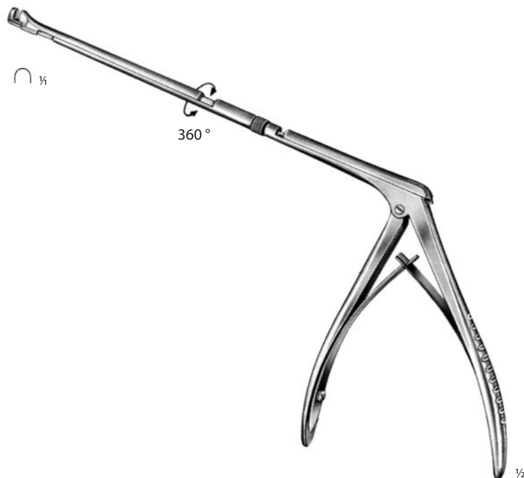
HAJEK-KOFFLER 116 91 0589 délka ramene 16,0 cm length of arm 16.0 cm
