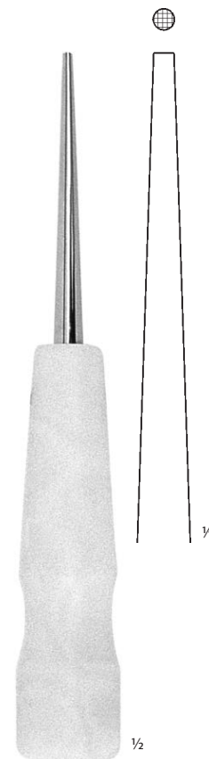
Zatloukač Punch 128 99 0015 21,0 cm Ø 1,5 mm
