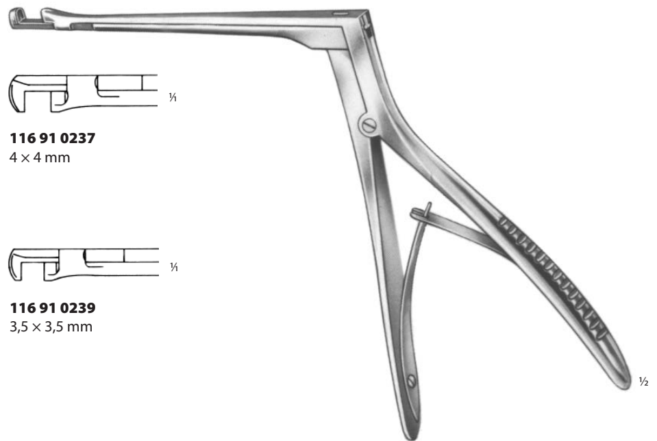
HAJEK-KOFFLER délka ramene 14,0 cm length of arm 14.0 cm
