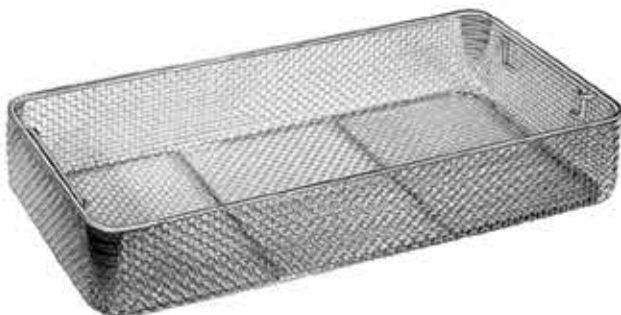
L(mm) 540 B(mm) 255 H(mm) 50 SK 307/05
